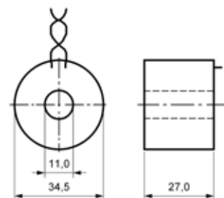
Elektronik-Stromwandler STWA 1 S
